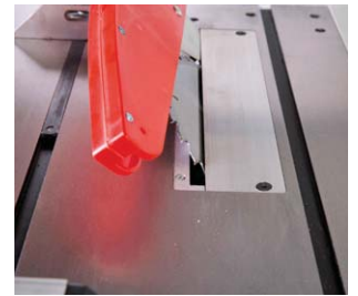
Sägeblattschwenkung von 90° bis -45° nach links
